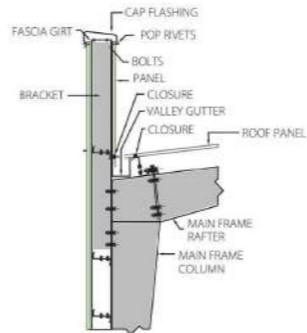
Parapet Fascia
